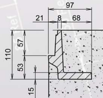
Typ Frame Section
